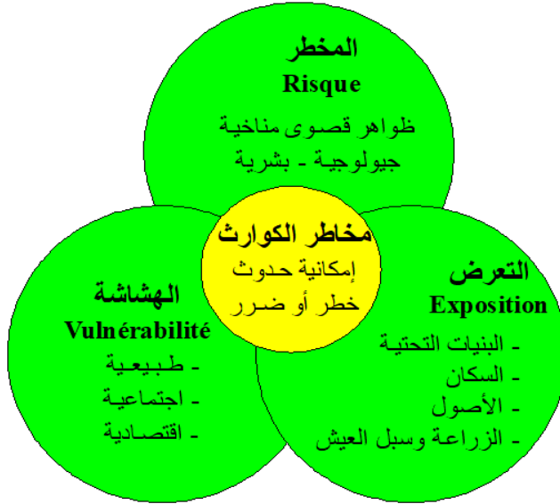
الشكل 1 - المفاهيم الأساسية المرتبطة بمخاطر الكوارث
