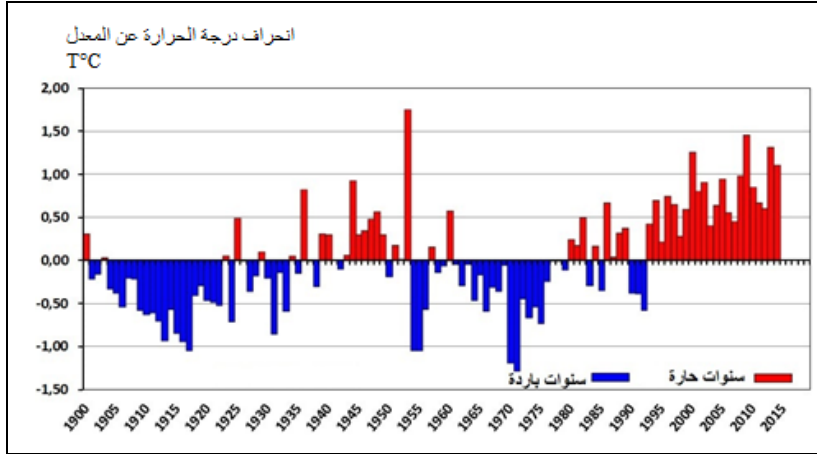
الشكل 2 - تطور انحراف معدل درجة الحرارة بالمغرب بين 1900 و 2015
