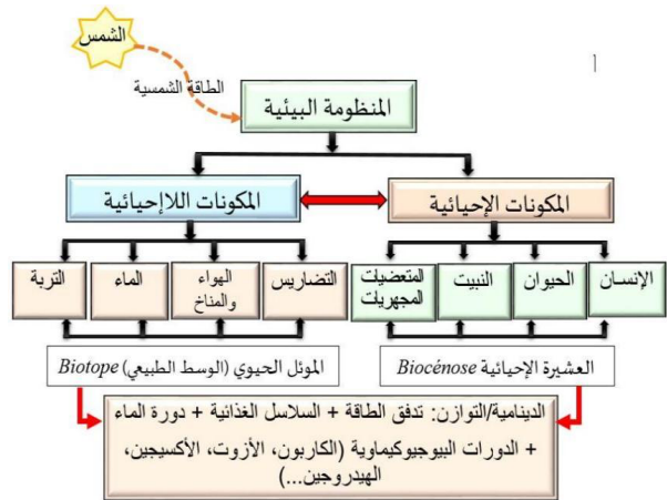
الشكل 2 - مكونات المنظومة البيئية وأسس توازنها
