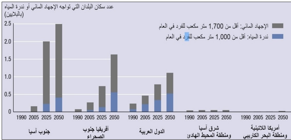
الشكل 1 - تطور الاجهاد المائي حسب اختلاف المناطق الجغرافية العالمية
