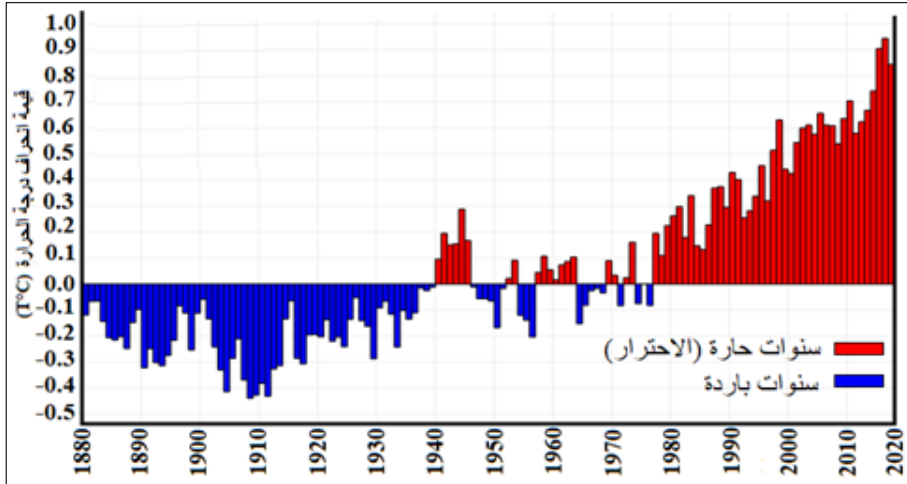
الشكل 1 - تطور انحراف متوسط درجة الحرارة في العالم بين 1880 و 2020
